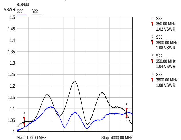
VSWR (BN 818433): S22 S33
