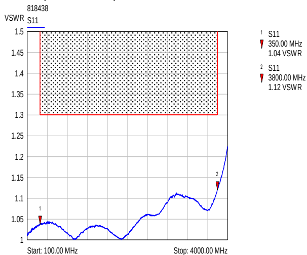
VSWR (BN 818438): S11
