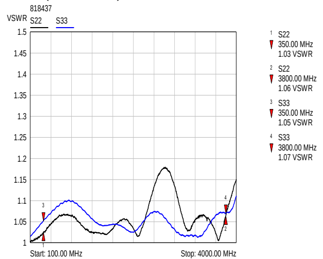
VSWR (BN 818437): S22 S33
