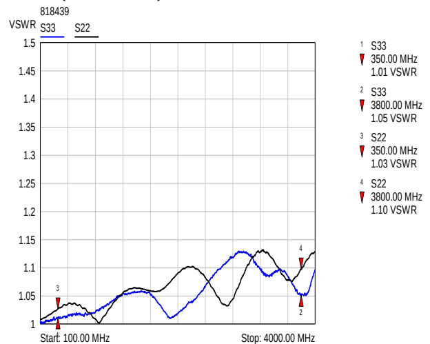
VSWR (BN 818439): S22 S33
